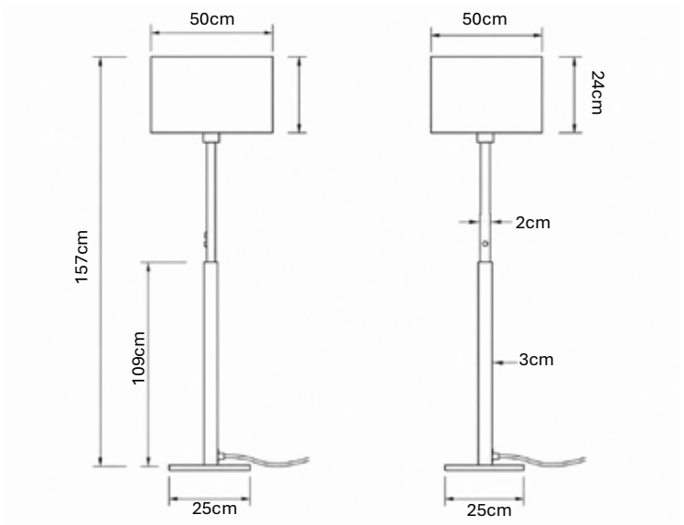
Technische Zeichnung Technical Drawing
